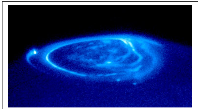
Figura. 02. NASA imagem de Júpiter Aurora Boreal em UV. Telescópio Espacial Hubble.
